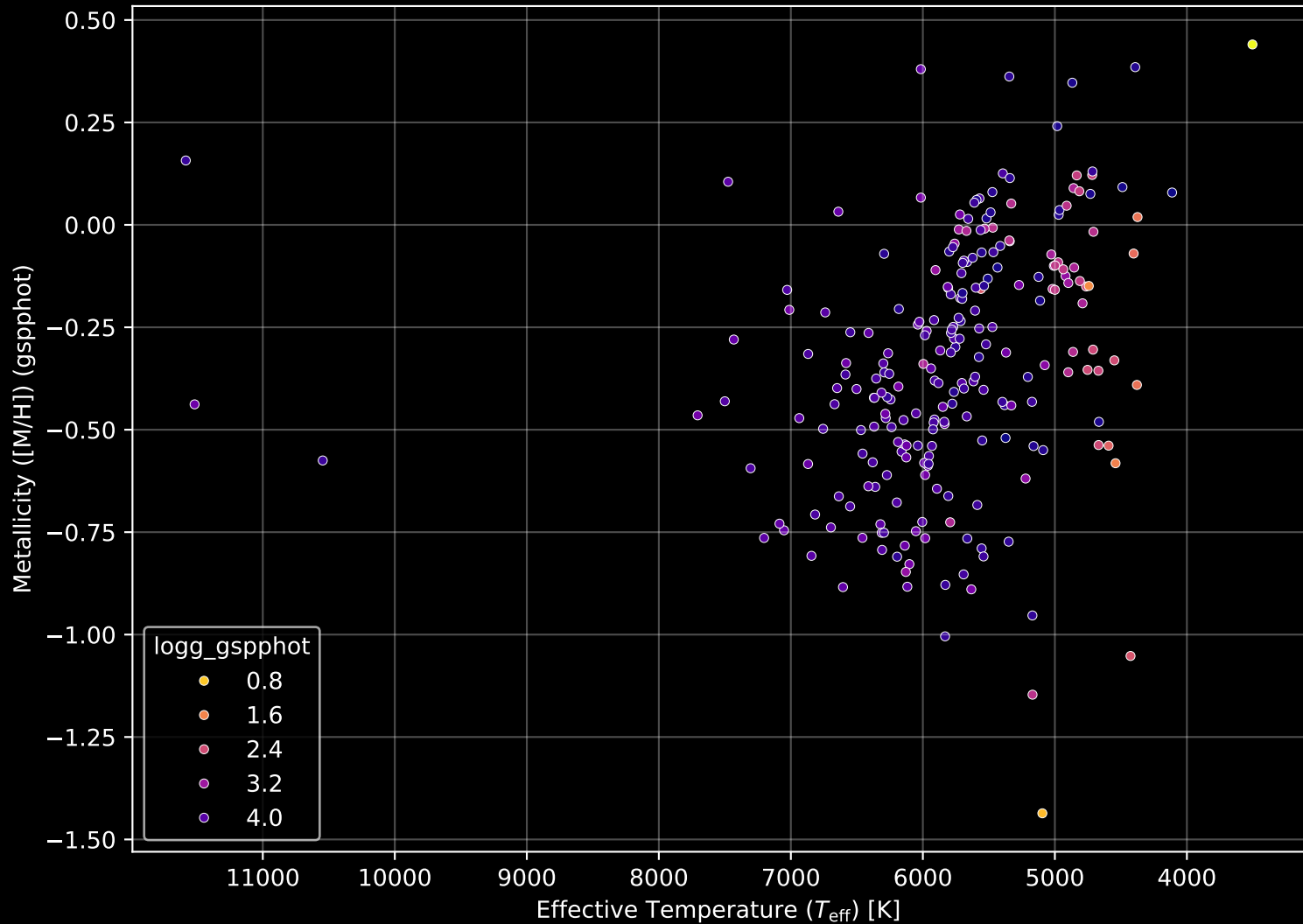
GALAH DR4 Field: [7167] Stellar Population Parameters (n= 239)
